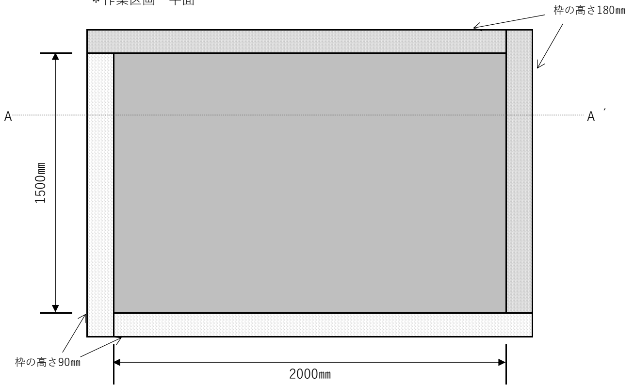
*作業区画 平面
