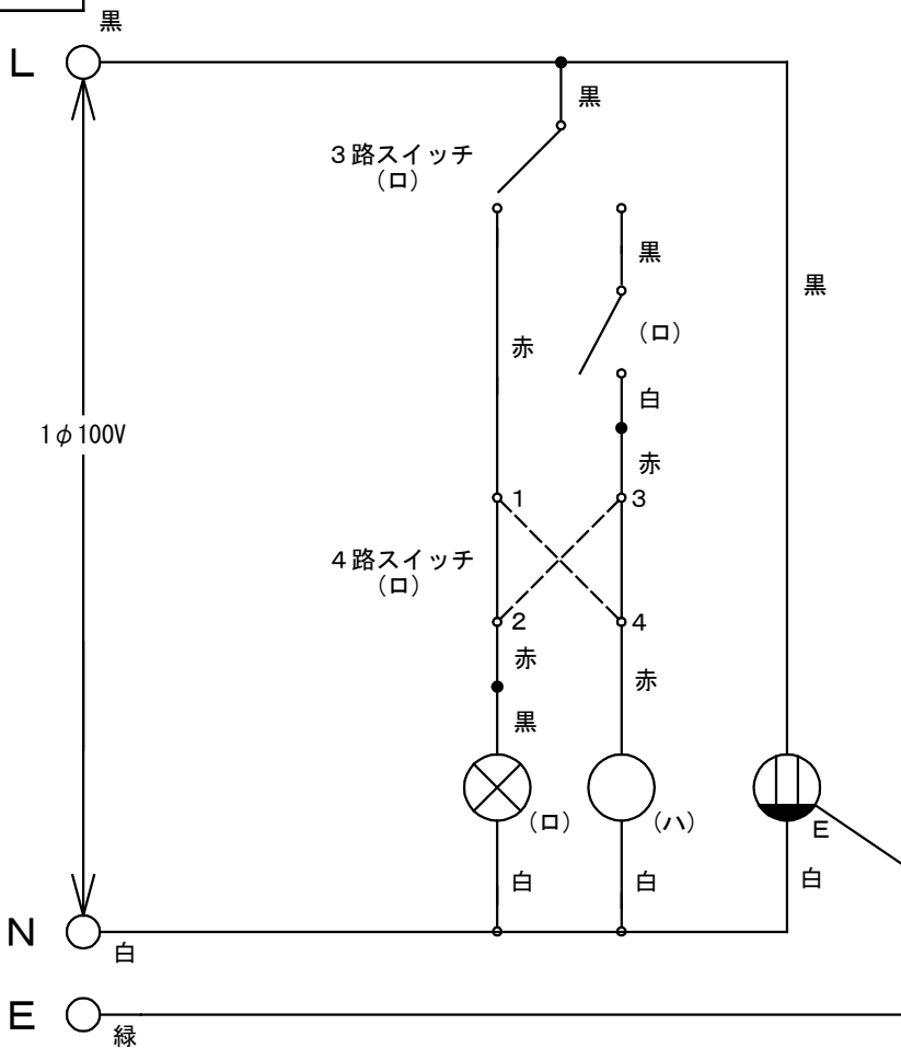
回路②
