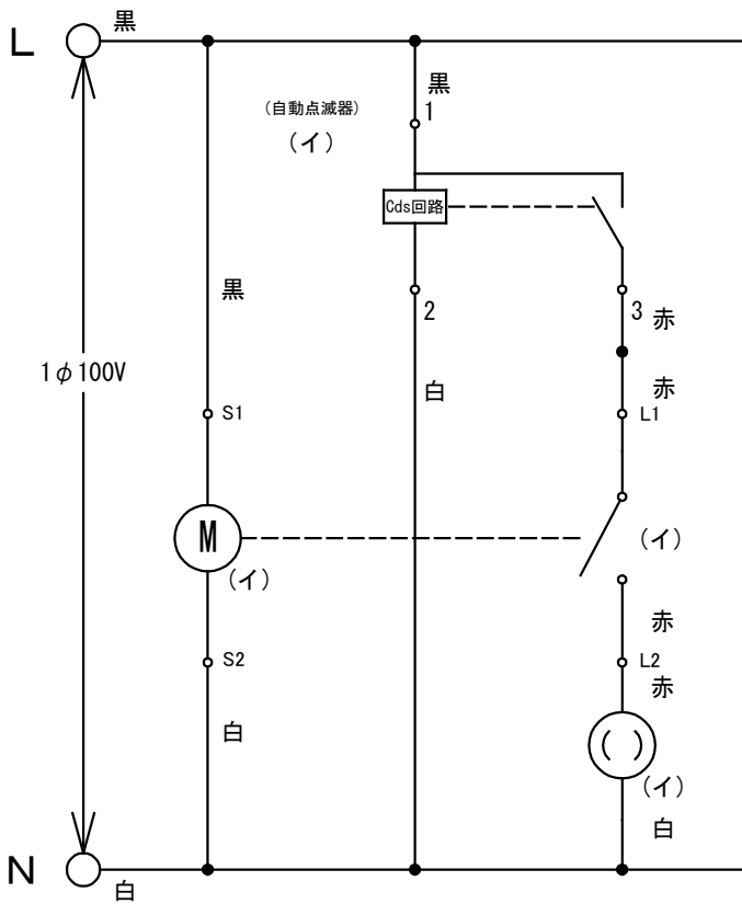
回路②
