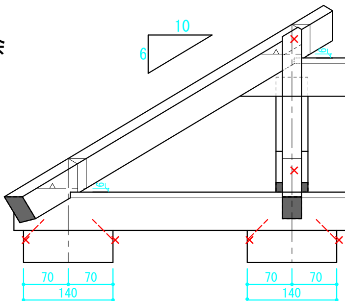
正面図
