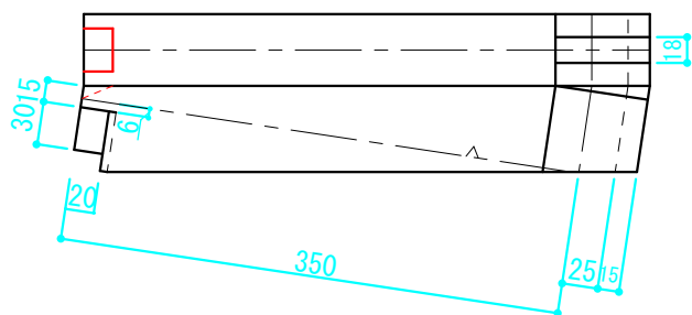
③登りばり 詳細
