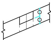
隅木側面 たる木大入れ取り合い
