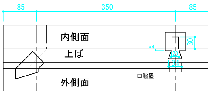
② 桁 詳細
