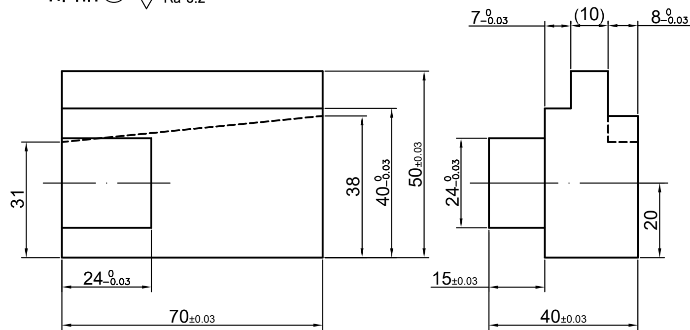
部品② \sqrt{\text{Ra } 3.2}
