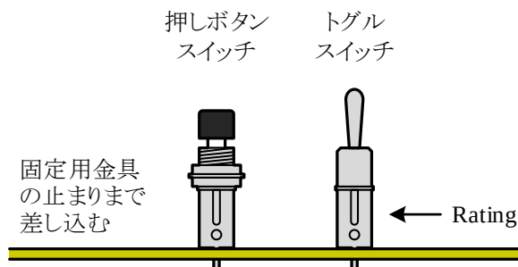
図8 スイッチの向きと取付け方
