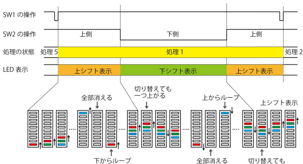
フルカラー10バーLEDの表示例
