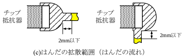
図 2 2 チップ抵抗器のはんだ付け基準
