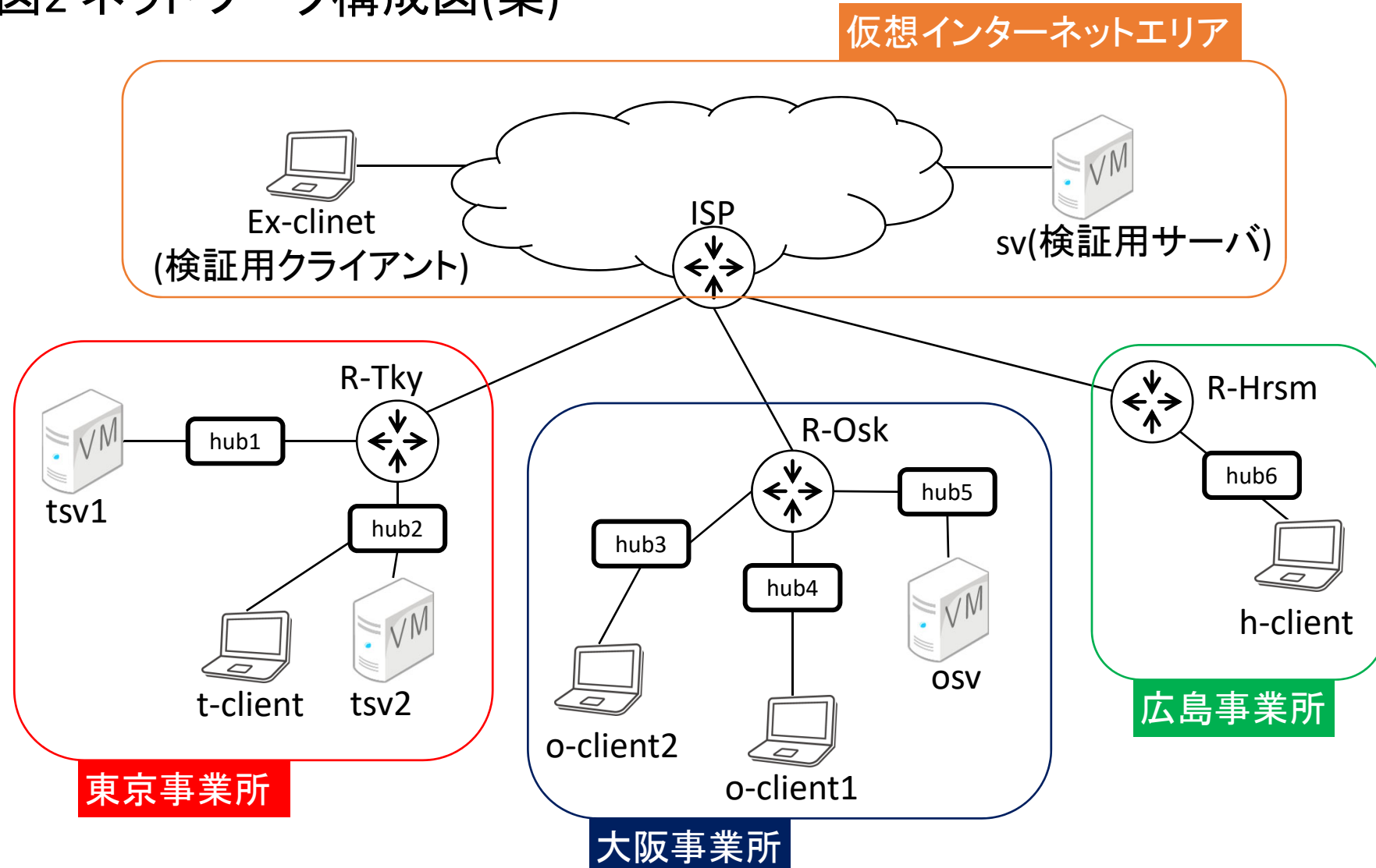
図2 ネットワーク構成図(案)
