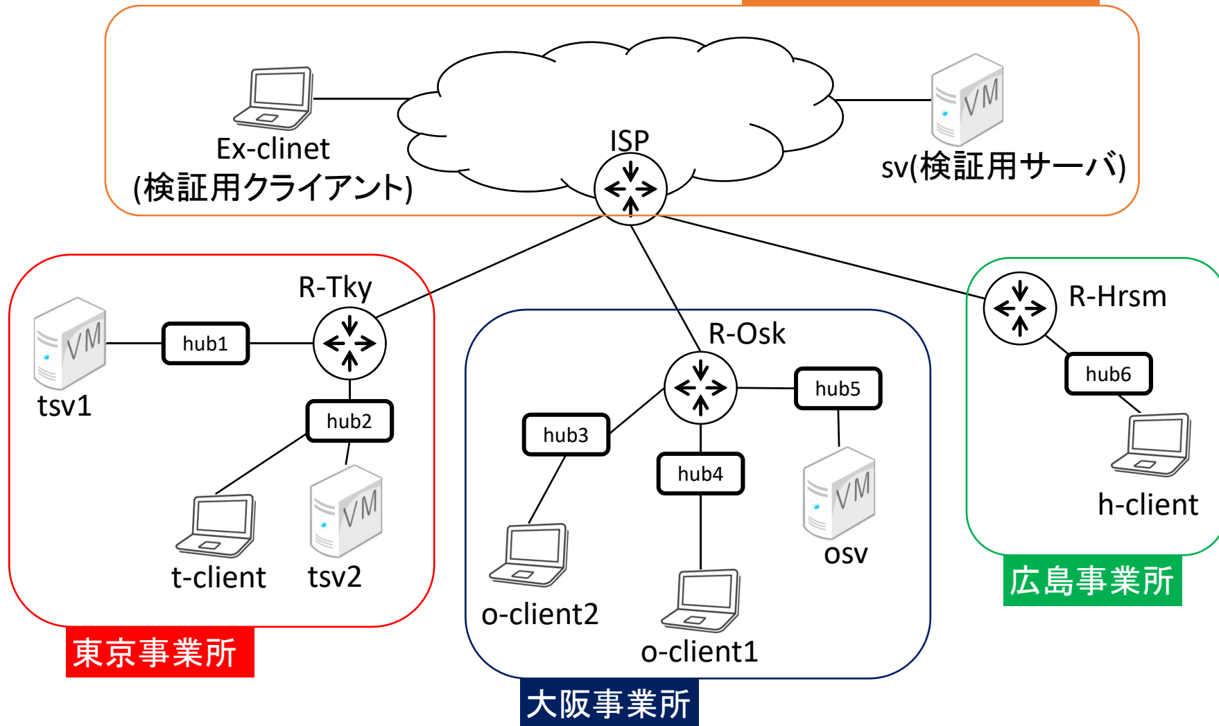
図2 ネットワーク構成図(案)
