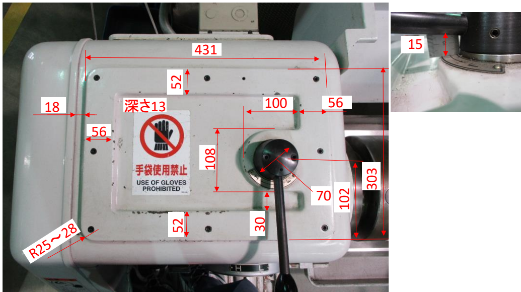
図3 主軸台
