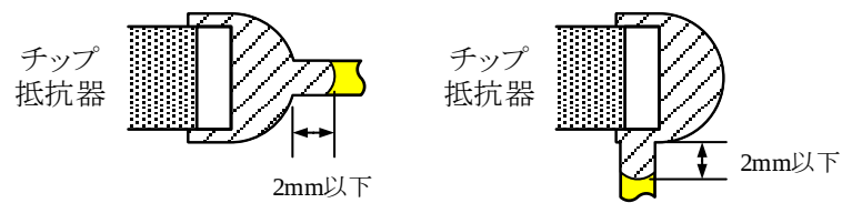
(c)はんだの拡散範囲 (はんだの流れ) 図 2 2 チップ抵抗器のはんだ付け基準
