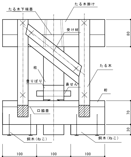
正面図
