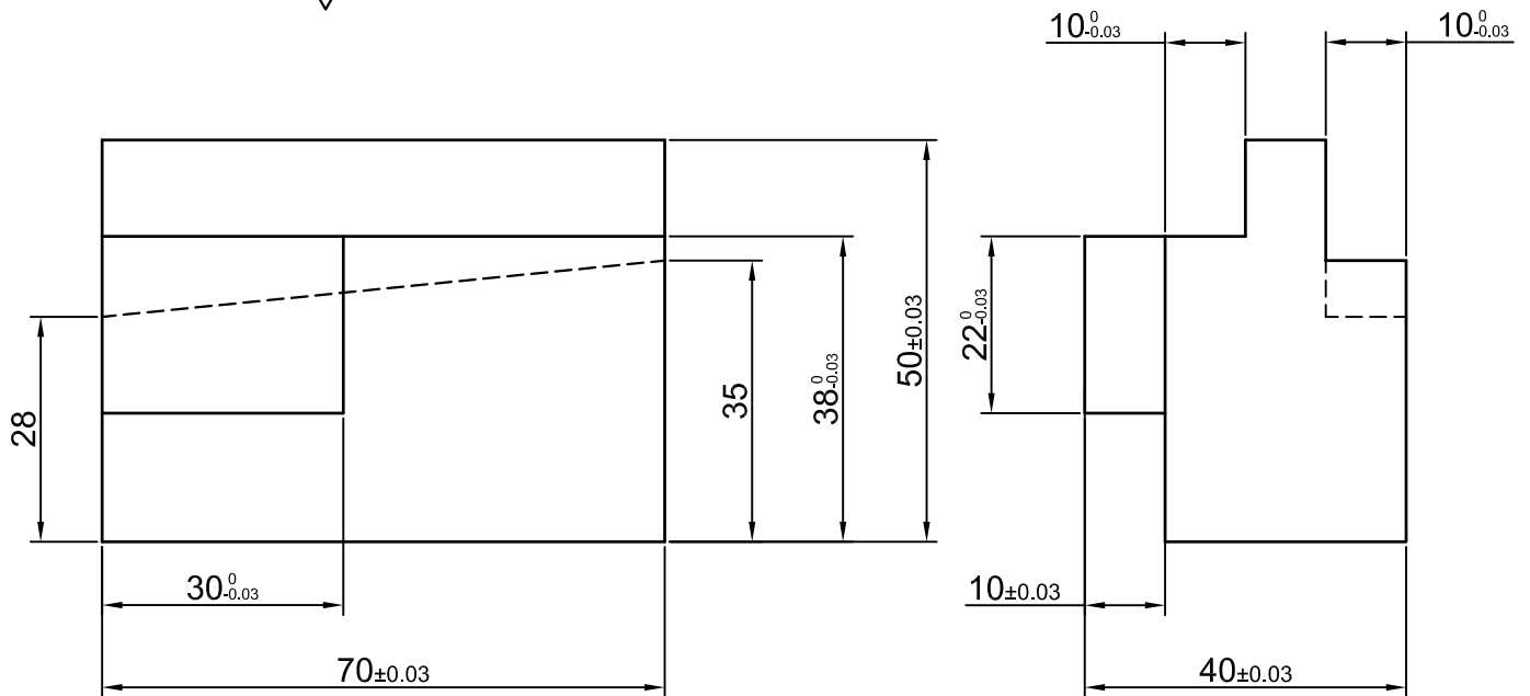
部品② \sqrt{\text{Ra 6.3}}
