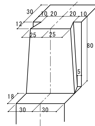
柱のたる木 掛け 取合い 詳細
