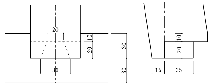
側面図
