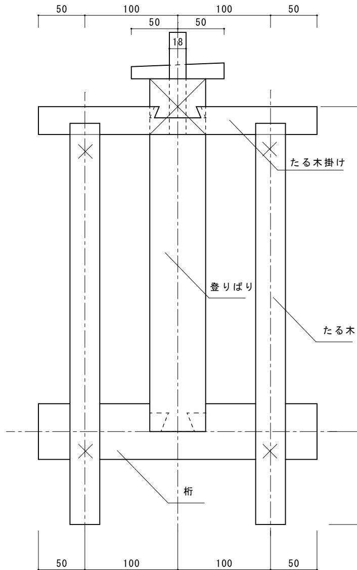
平面図
