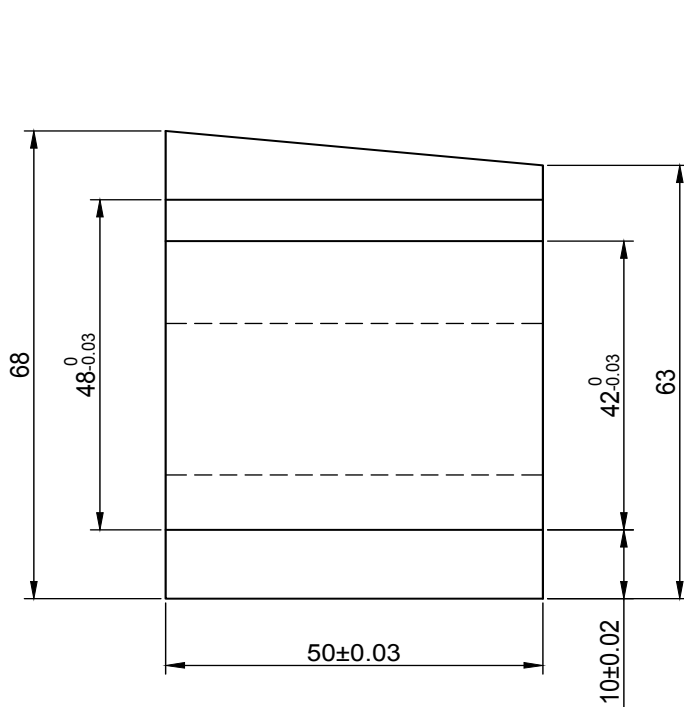
部品 ① \sqrt{Ra\ 6.3}
