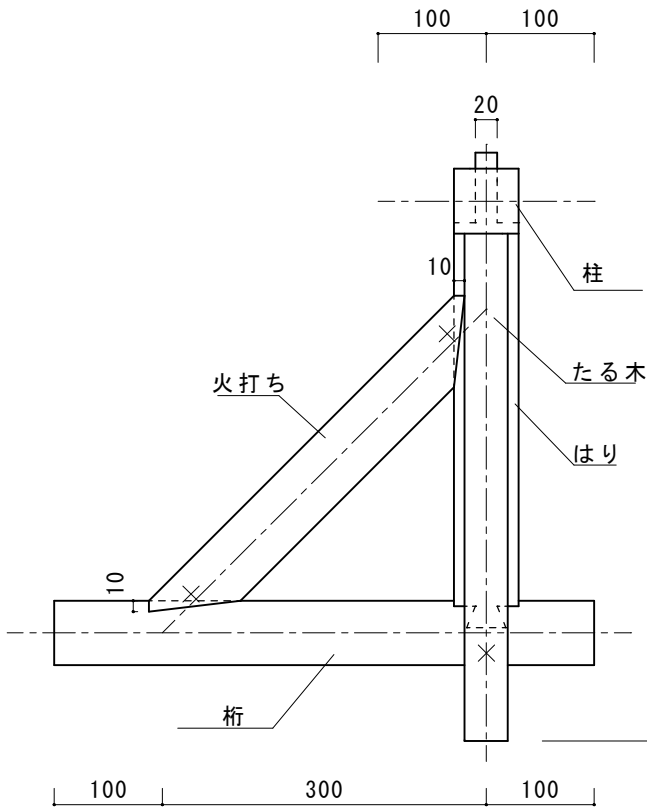
平面図
