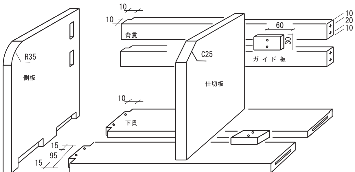
分解図
