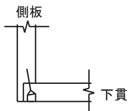
くぎ打ちだぼ埋め（左側）
