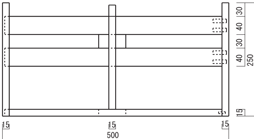
三面図
