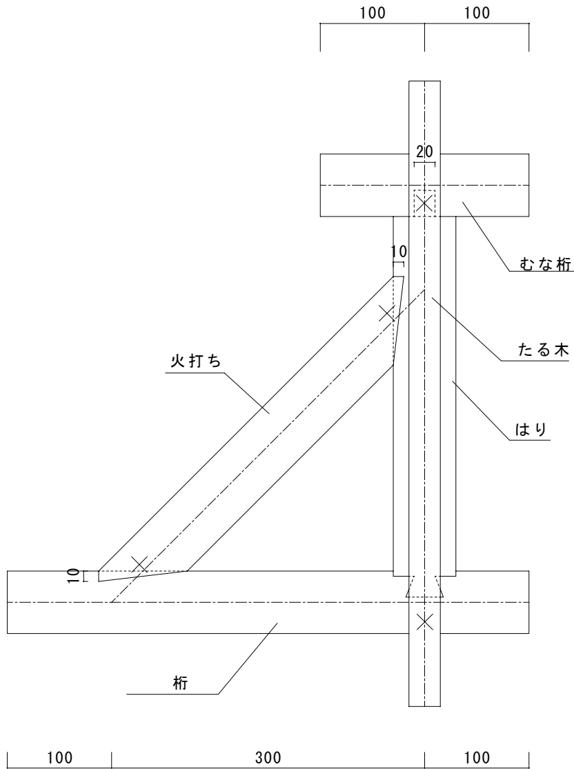
平面图
