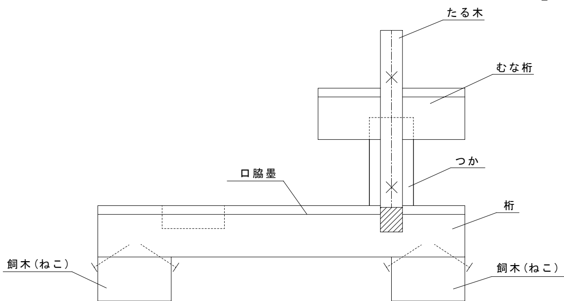
正面図
