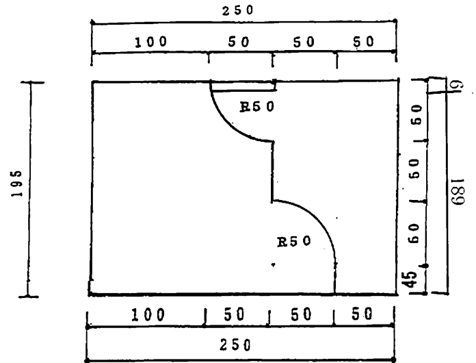
左側面図
