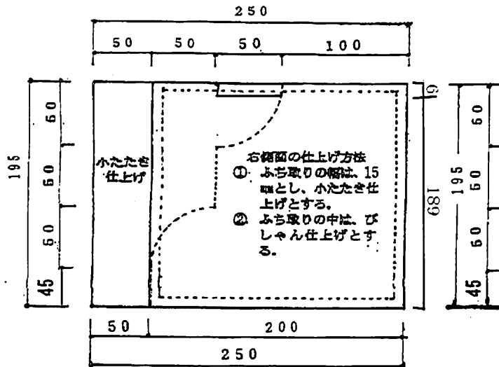
右側面図
