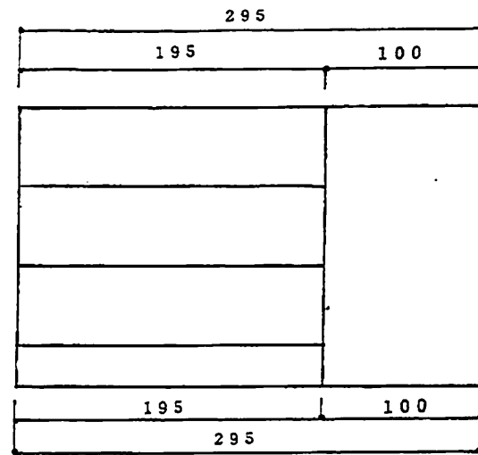
正面図
