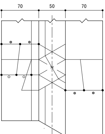
④ 桁詳細図ねじ組
