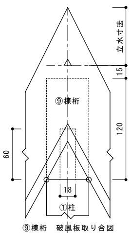
⑨棟桁 破風板取り合図
