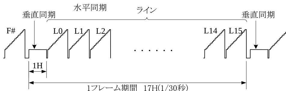
図 8 コンポジット信号の構成
