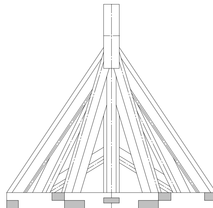
背面図
