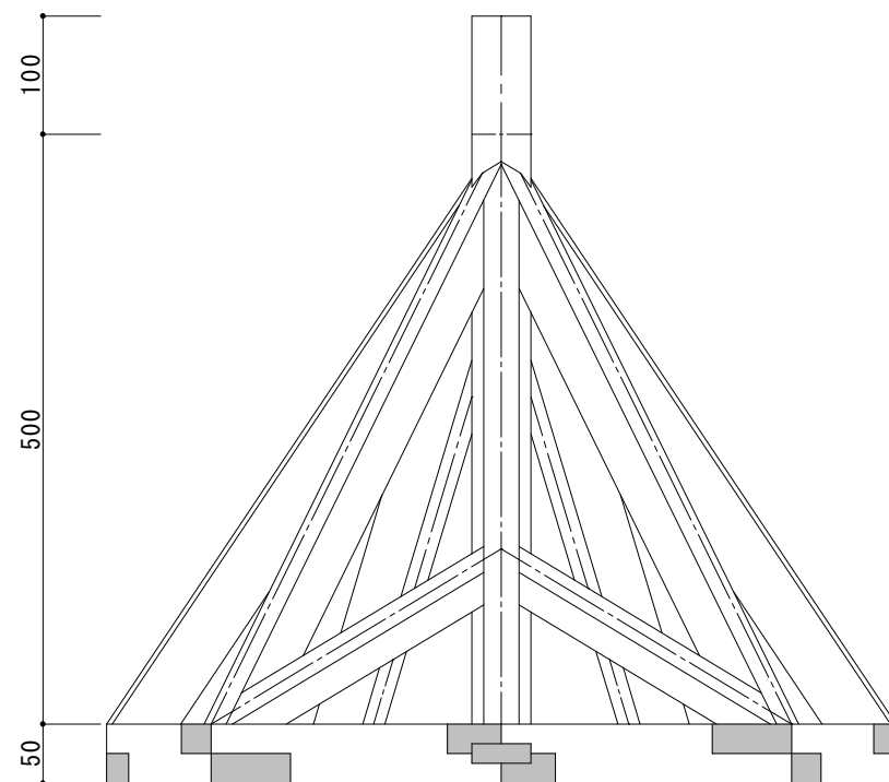
正面図
