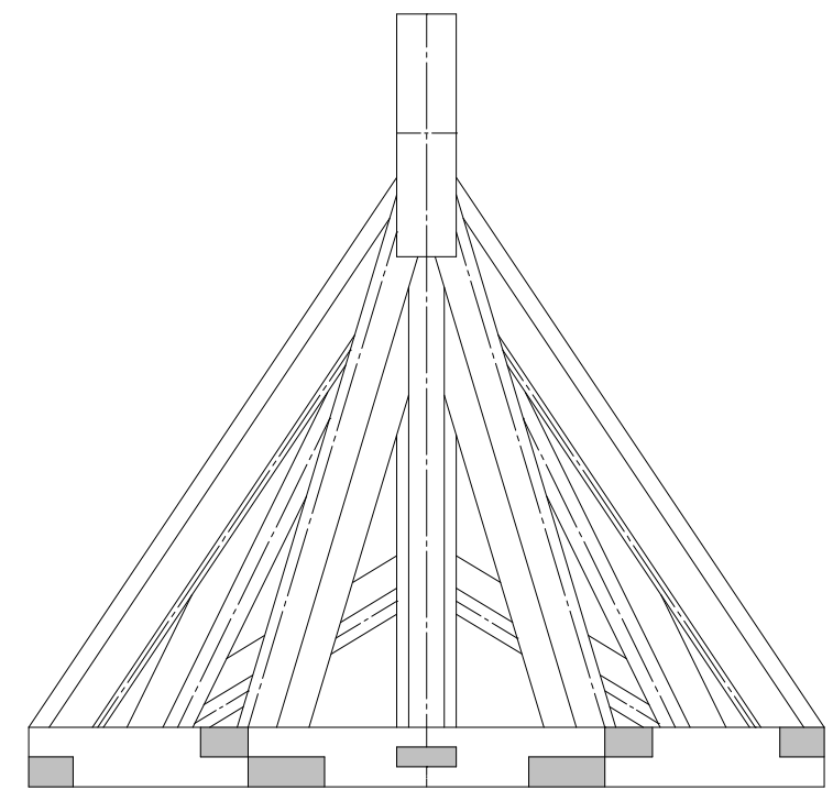
背面図
