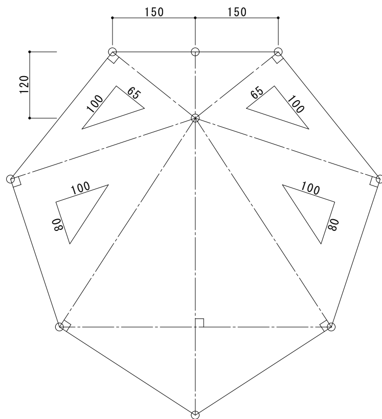
平面基本図
