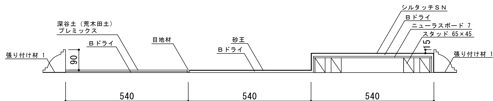
b-b' 断面図 S=1:10
