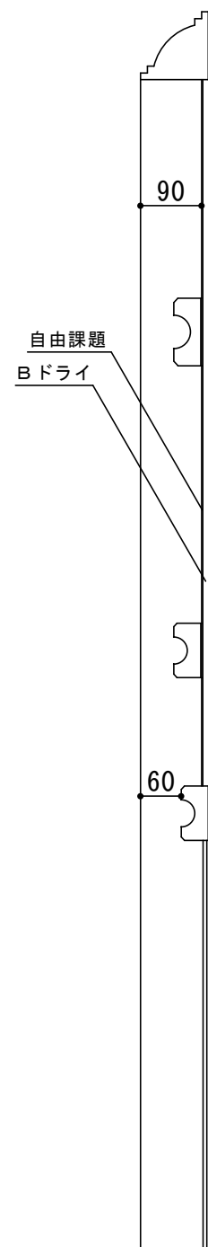
c-c' 断面図 S=1:10
