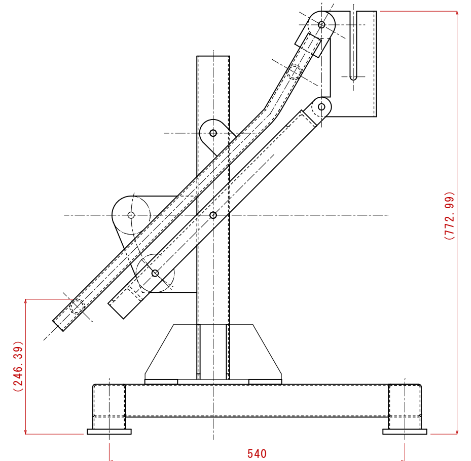
正面図（姿勢B）
