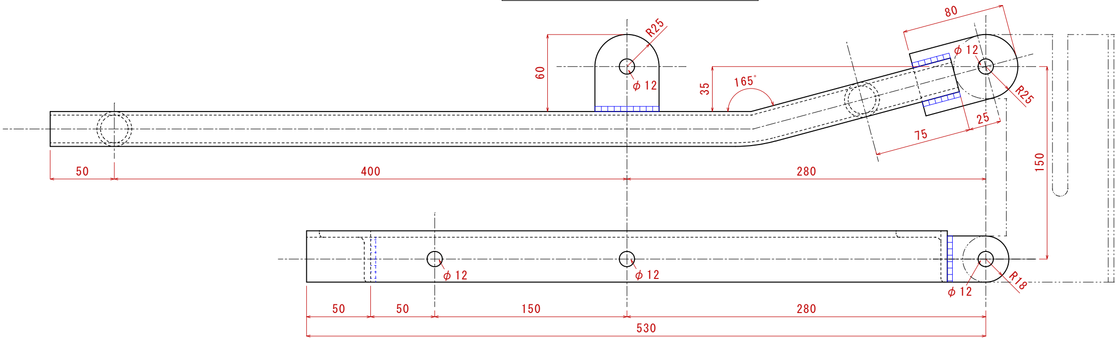
部品NO. 4正面図
