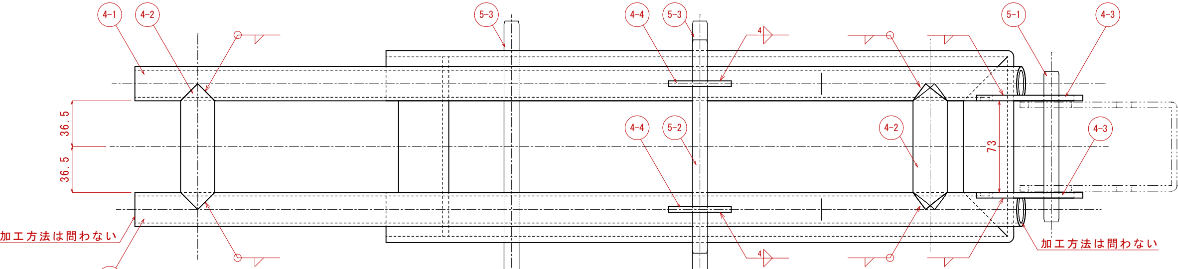
部品NO. 4・5 平面図
