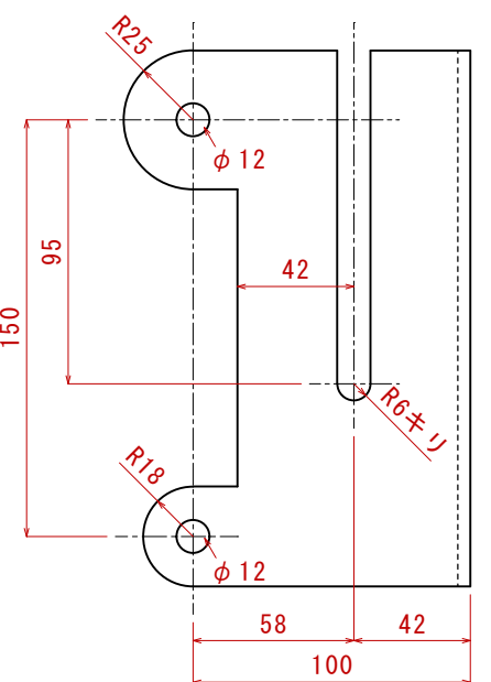
部品4-5 正面図
