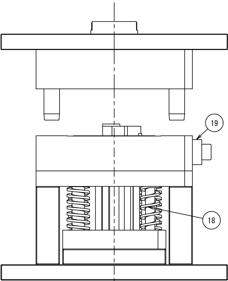
金型開状態側面 (1:1.5)
