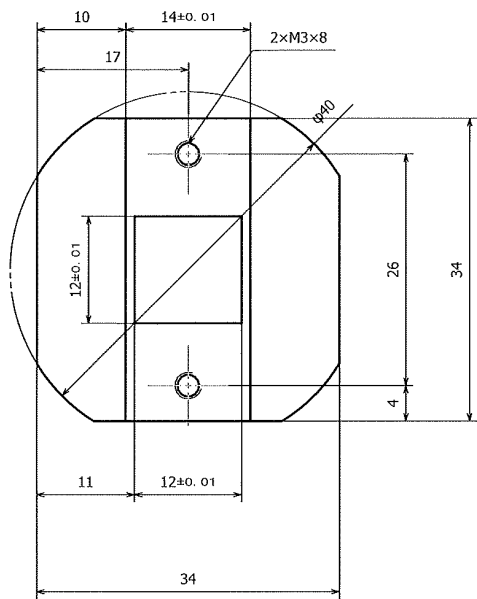
部品図
