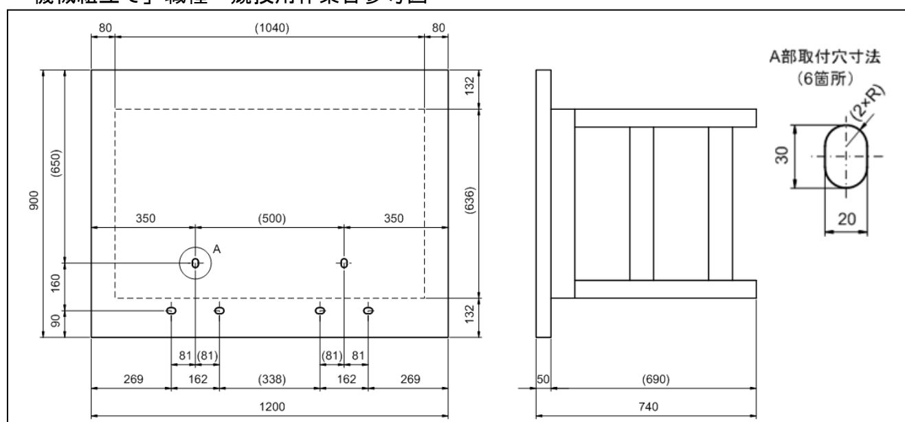
「機械組立て」職種 競技用作業台参考図
