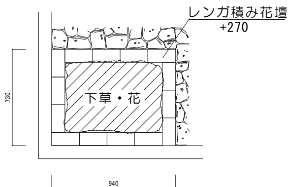
レンガ積み花壇平面図
