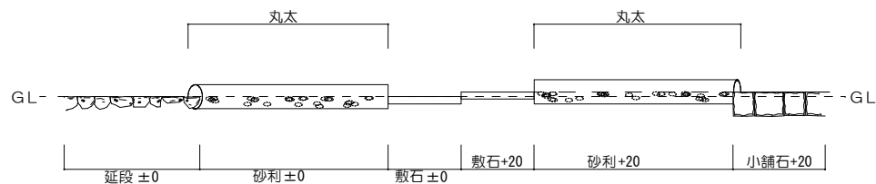
敷石部断面図
