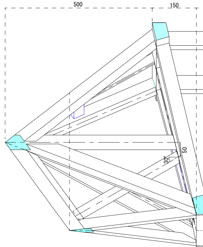
側面図
