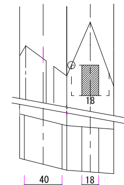
①柱・⑩棟木取合詳細図
