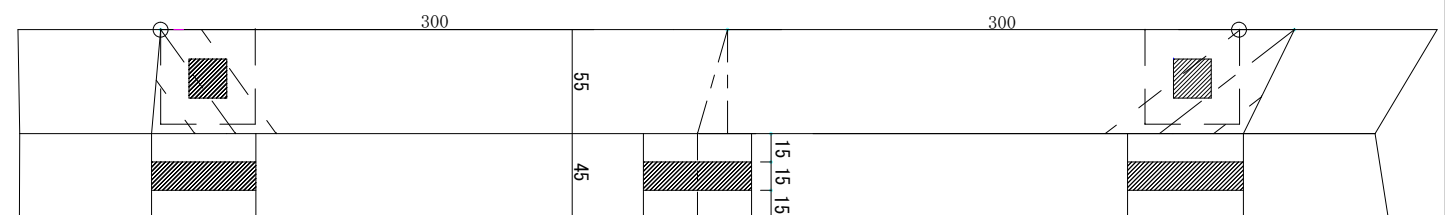
⑤桁・梁取合詳細図
