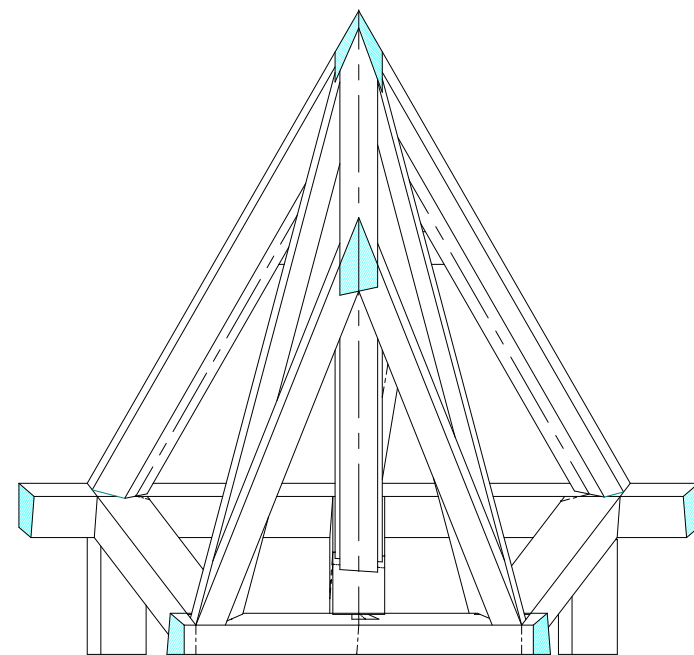
正面図
