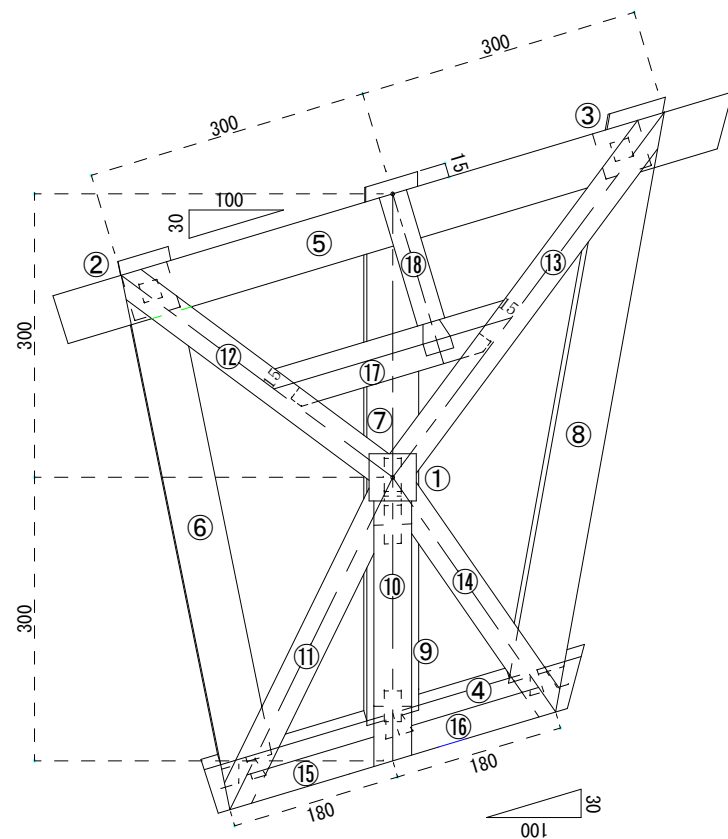
平面図
