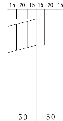
②③柱ほぞ詳細図
