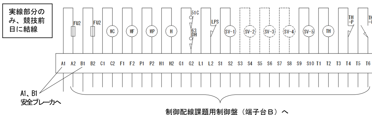
図 2 端子台 C 配線接続図
