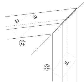
②① ②② 広小舞取合い図
