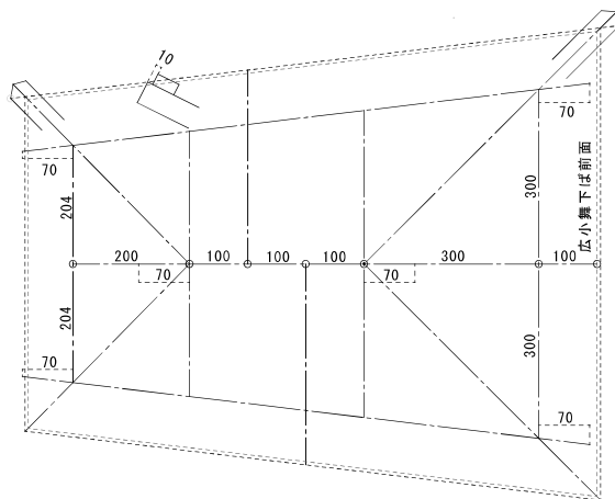
平面基本寸法図
