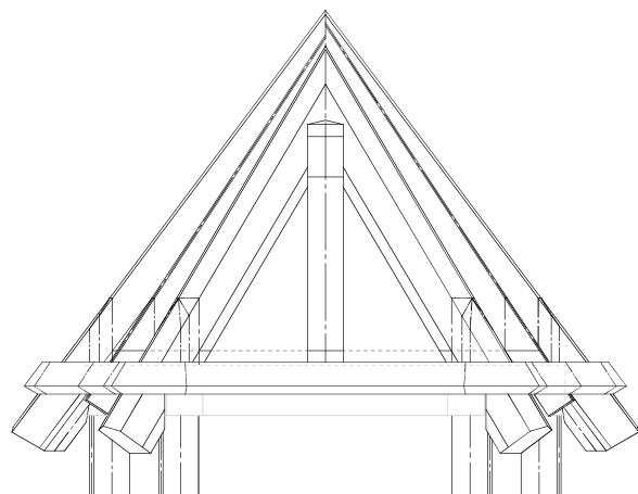
正面図
