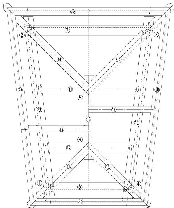
平面図
