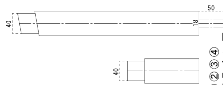
②① ②② 広小舞取合い図
