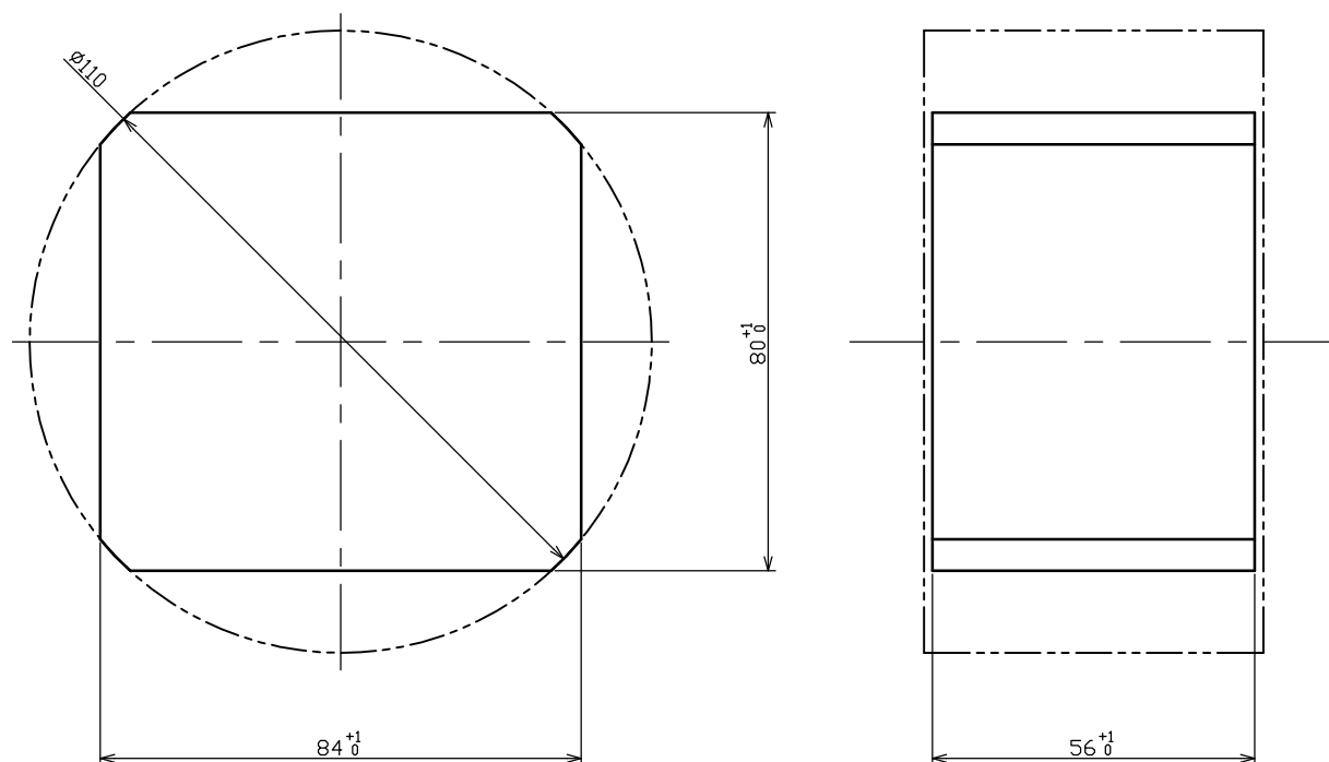
部品① \phi 110 \times 60
