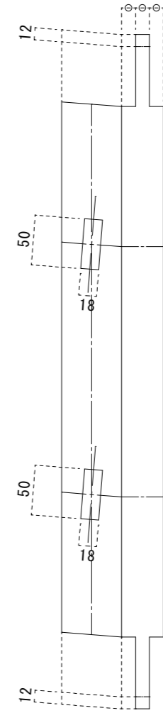
⑪ 梁・柱取合い詳細図
