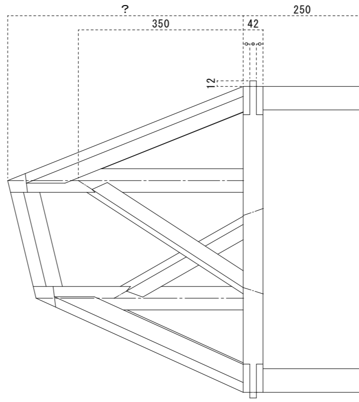
側面図
