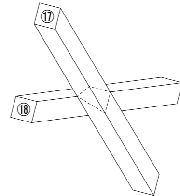
筋かい詳細図
