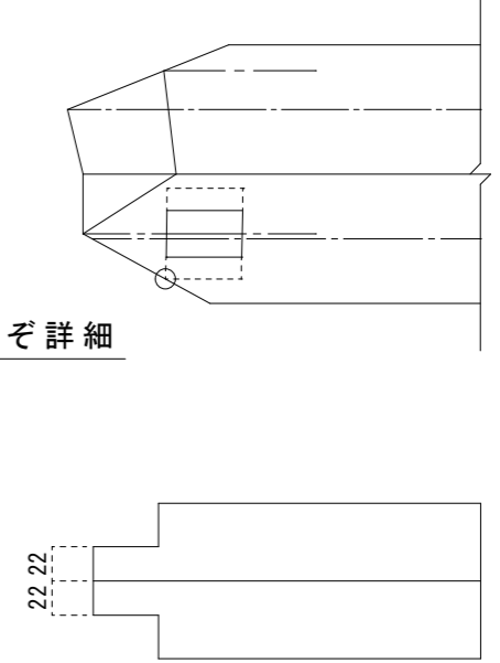
⑤ 柱・棟木取合い詳細図
