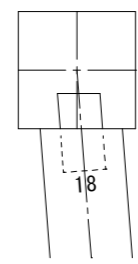
棟木ほぞ詳細
