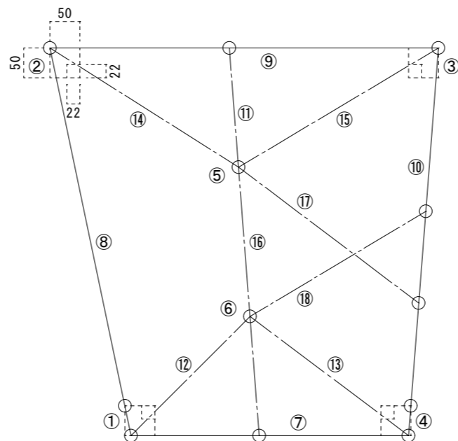
平面基本図
