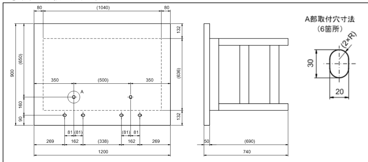
「機械組立て」職種 競技用作業台参考図
