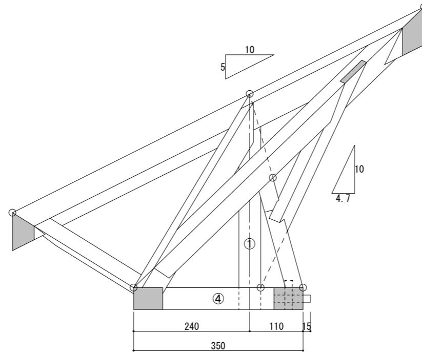
側面図
