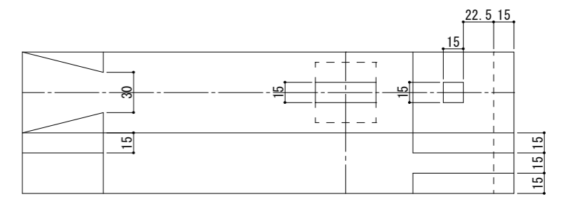
④梁詳細図
