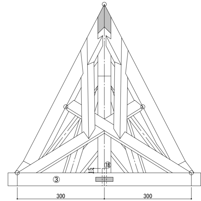
背面図
