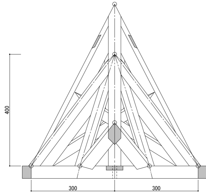
正面図
