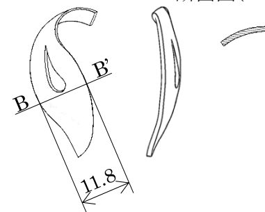
断面図(B-B')
