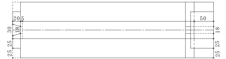
⑭ 梁 詳細図
