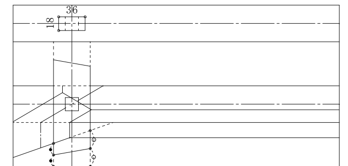
⑫ 桁下木ねじ組 詳細図
