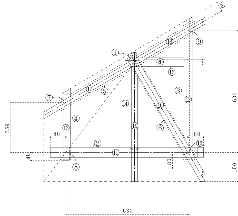
平面図
