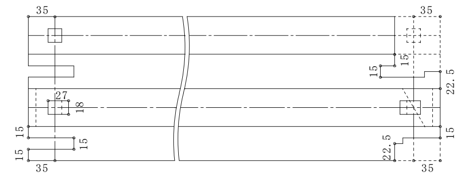
② 土台 詳細図
