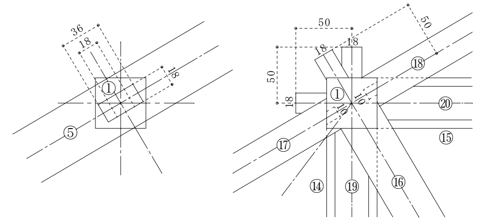
① 心柱根ほぞ 詳細図
