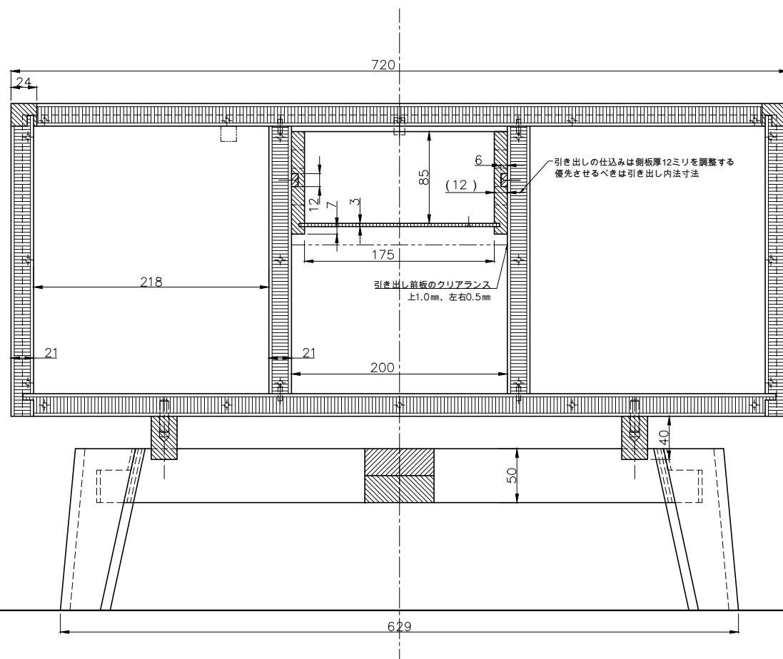
B-B断面図
