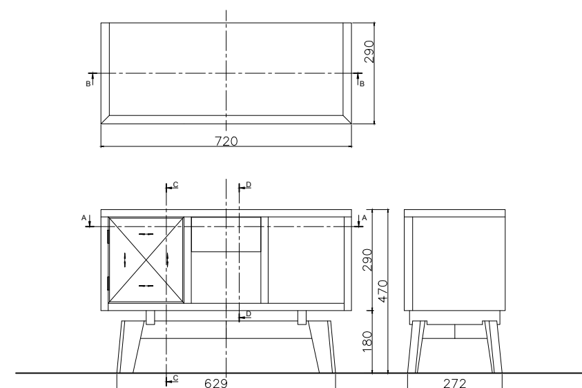
三面図
