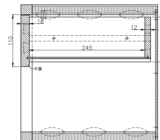
D-D断面図 ( 引き出し位置 )
