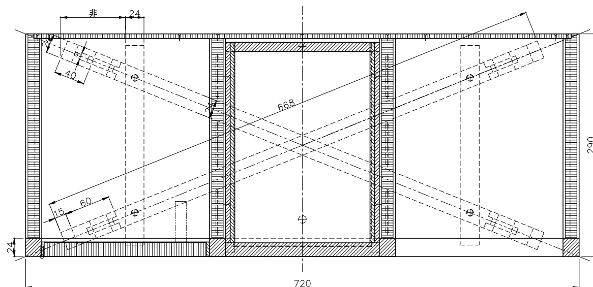
A-A断面図
