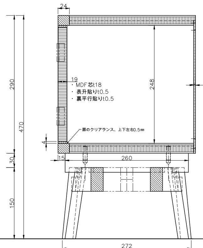
C-C断面図 ( 扉位置 )
