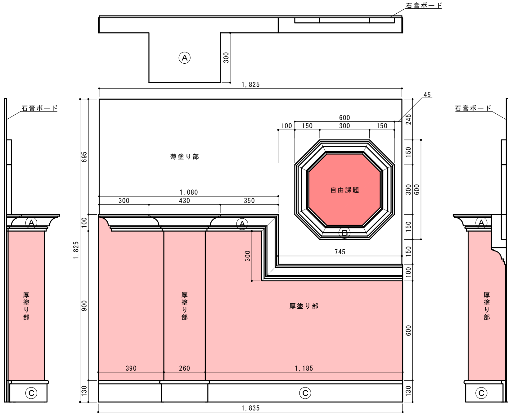
左官職種 1 - 1 競技課題図
