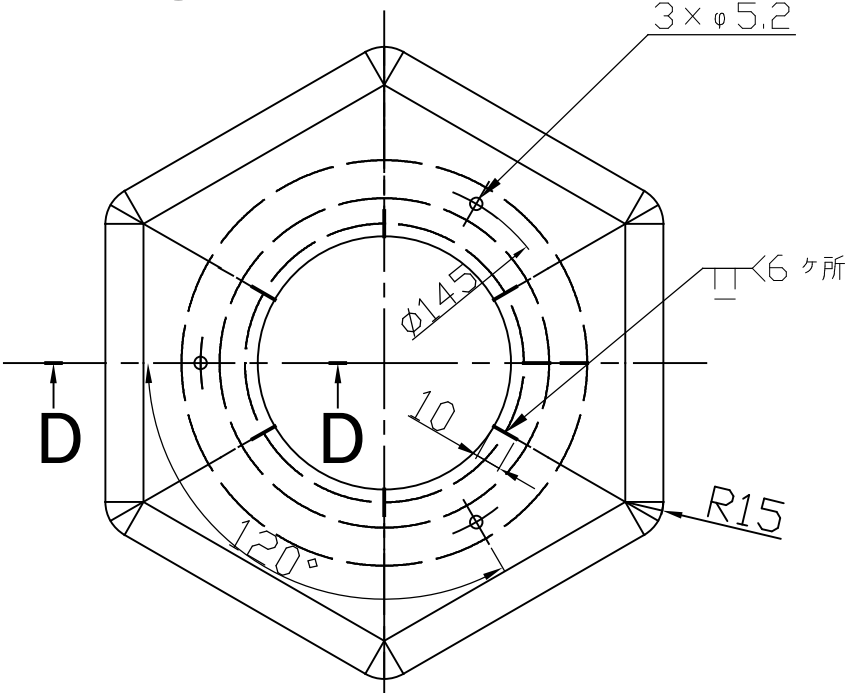
B-B矢視
