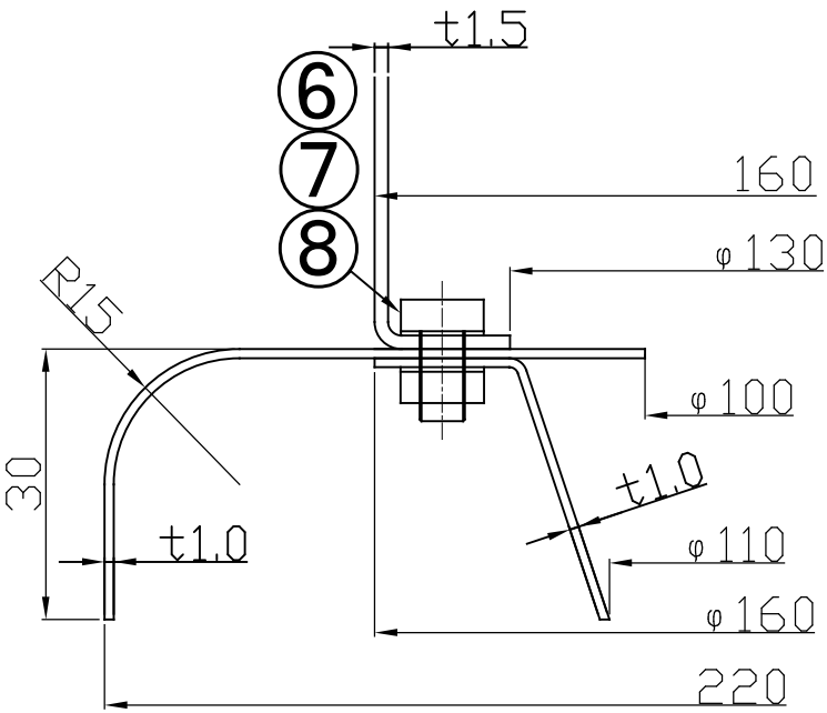
D-D断面
