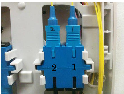
図3 光アダプタとコネクタ
