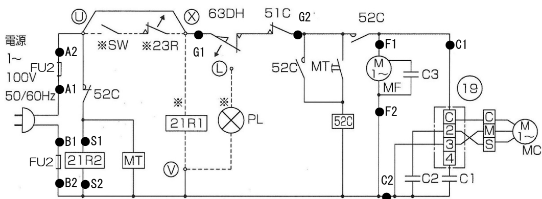
図 2 端子台 C 配線接続要領
