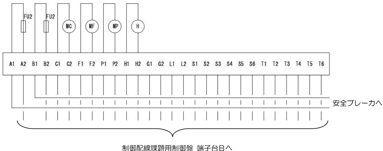
図 2 端子台 C 配線接続要領
