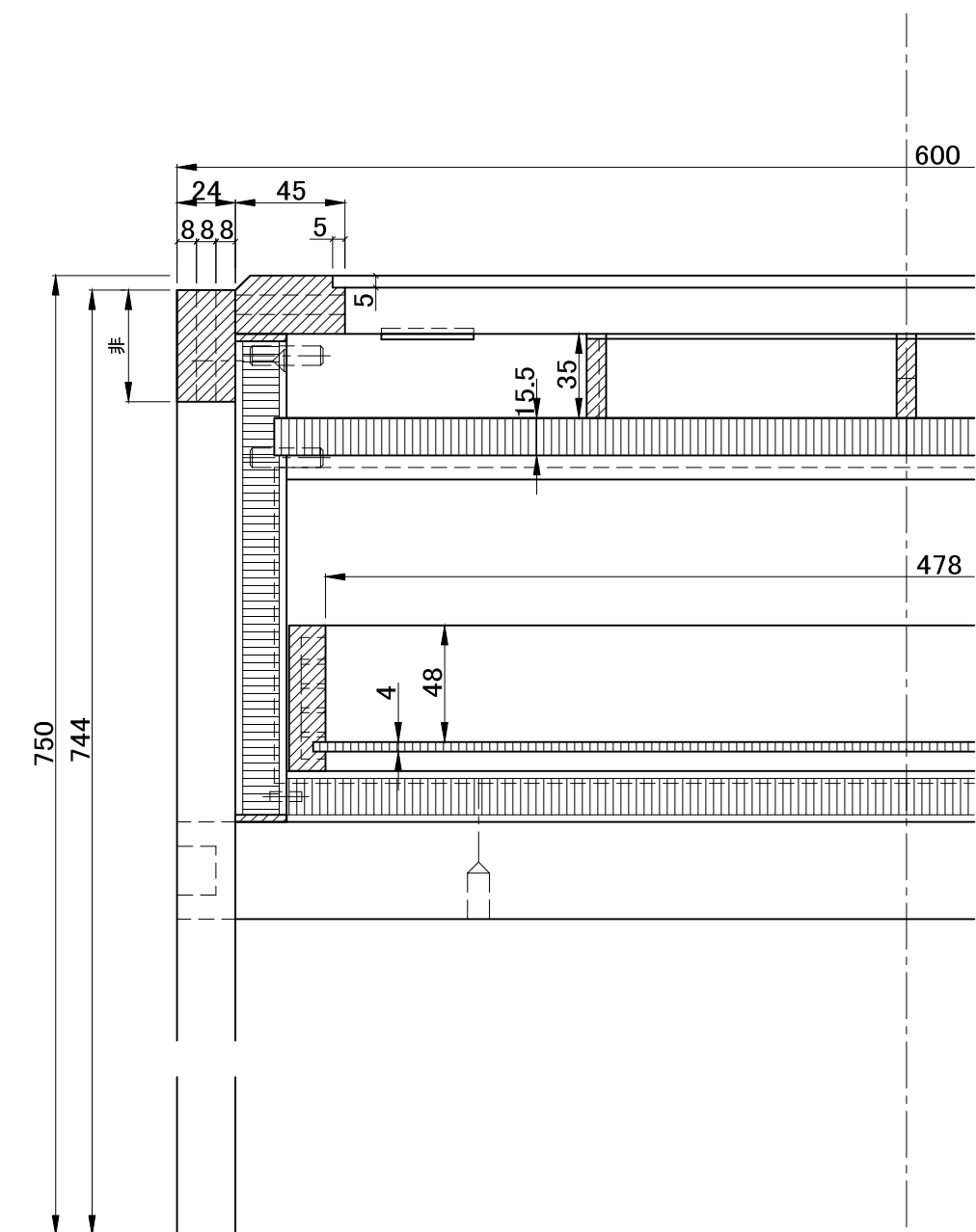
C-C断面
