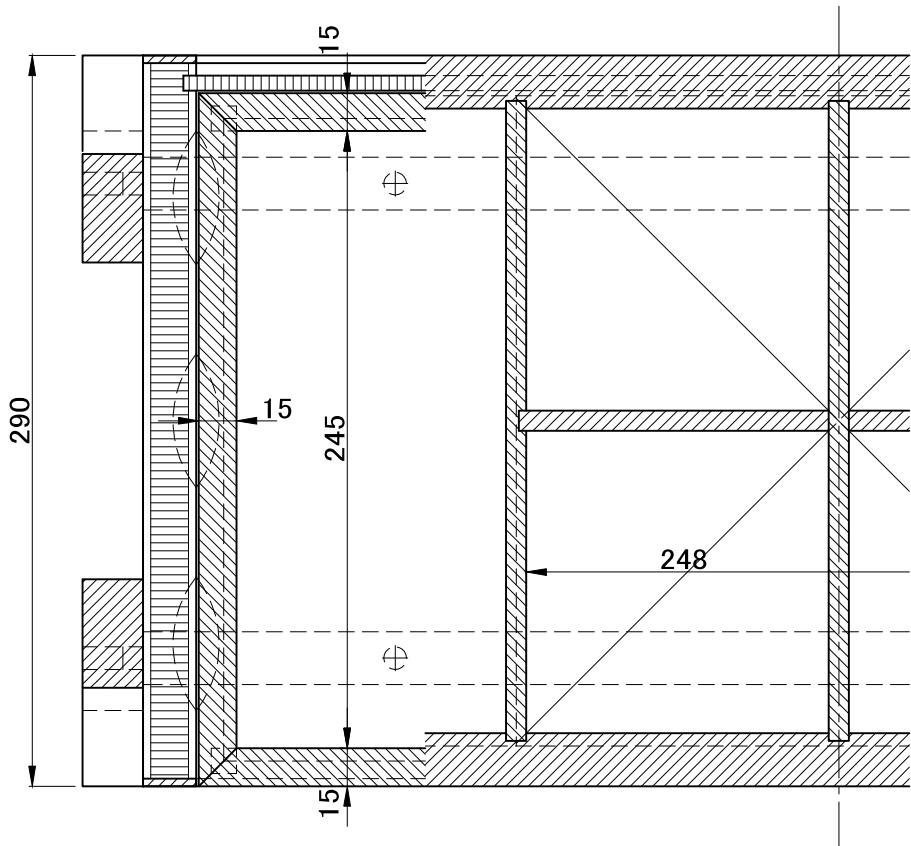
A-A断面
