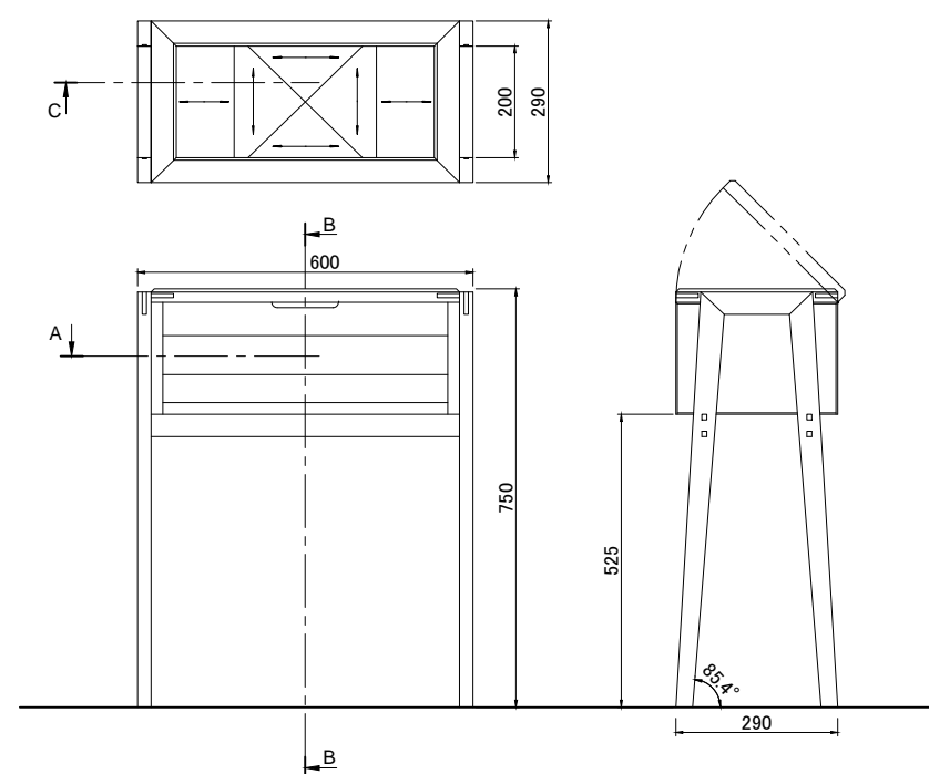
三面図
