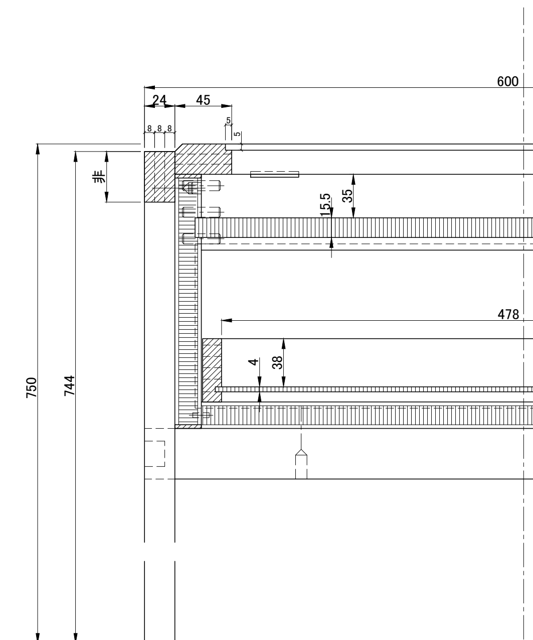
C断面
