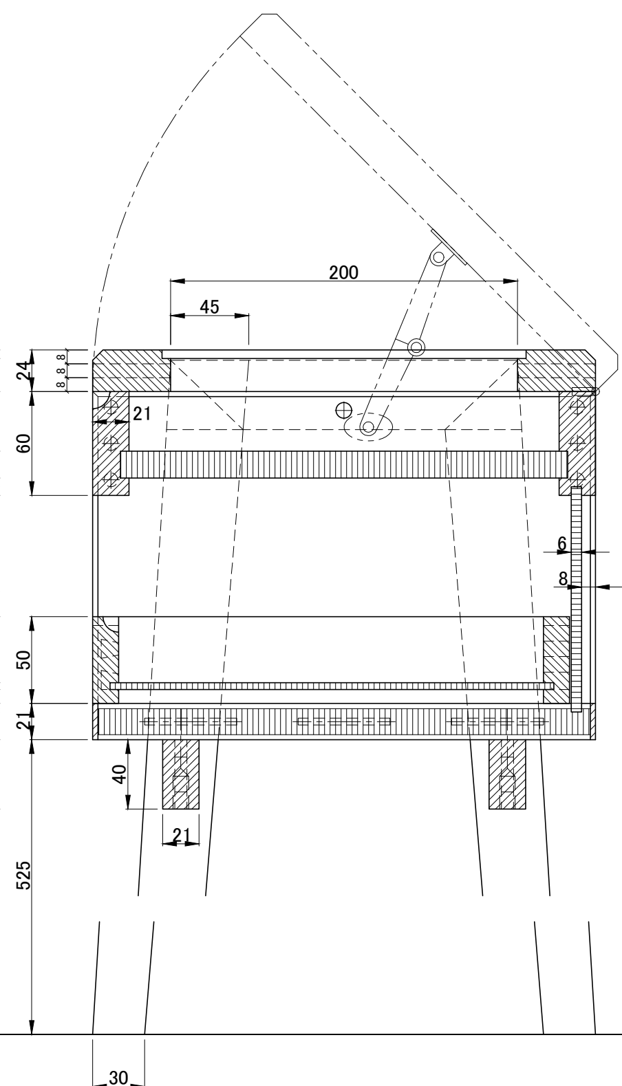
B-B断面
