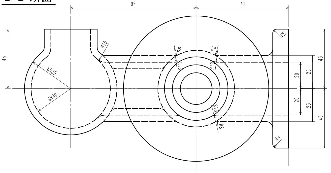
D-D 断面
