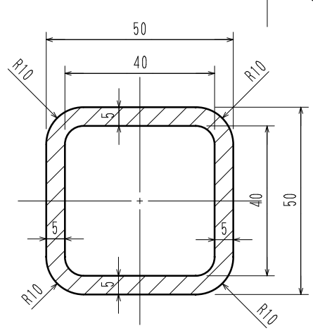
D-D 断面
