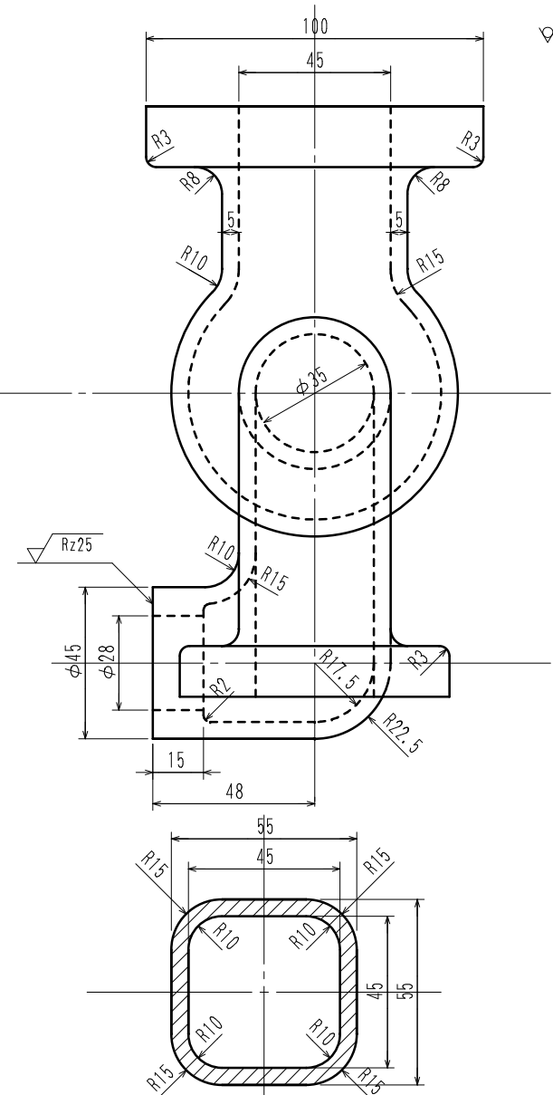
A-A 断面
