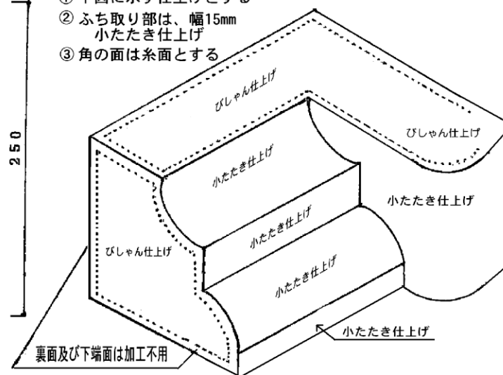
完成図
