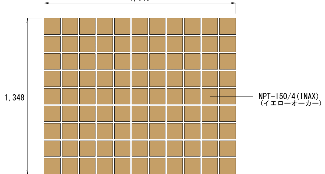
平面図 1,648
