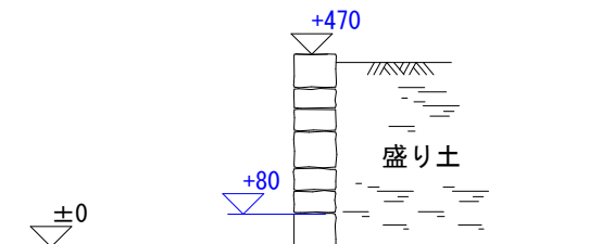
D ▲ ▲ D 断面図 S=1:20
