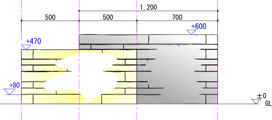
石積み正面図
