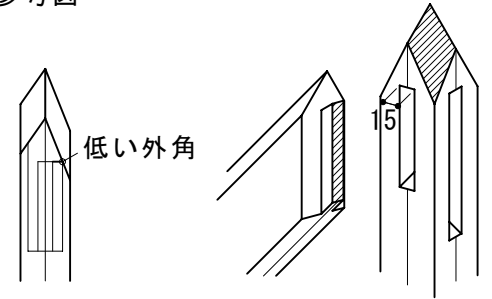
⑦柱・⑨隅木取り合い
