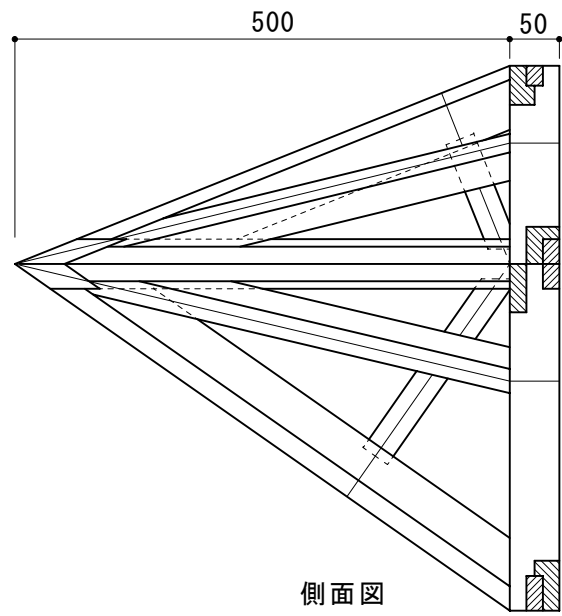
各部参考図
